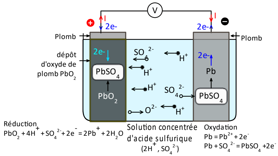
Schéma d'un accumulateur plomb-acide
